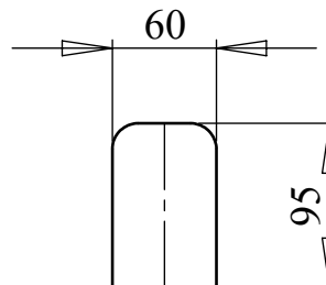
Внутренняя часть бампера Рис.1 Рекомендуемый вырез
